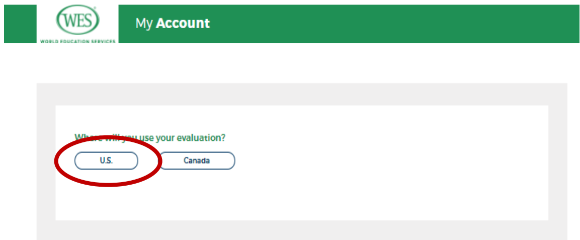
Fig. 3: Elegimos país.
